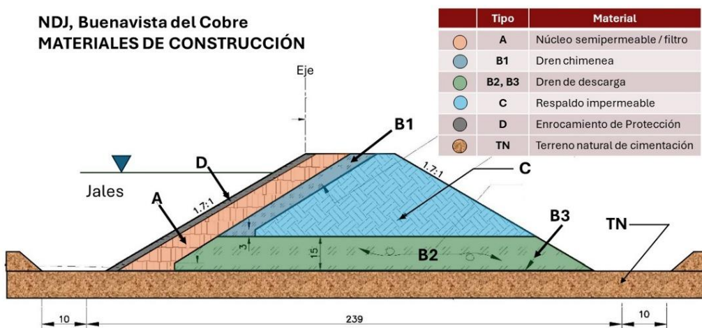
(b) Cortina flexible, filtrante y zonificada con respaldo impermeable.
