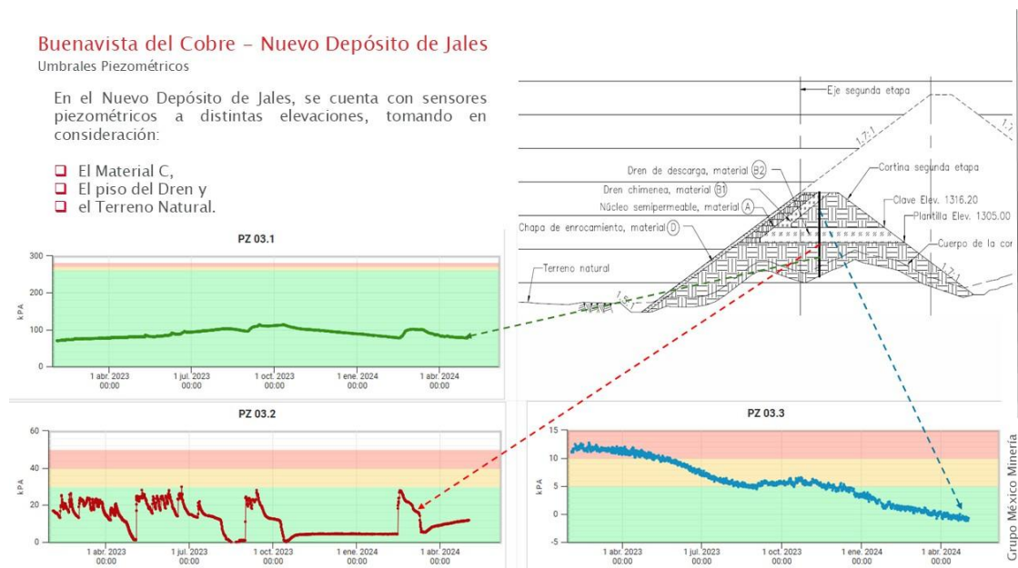
Ilustración 3. Instrumentación electrónica digital en tiempo real de la cortina del NDJ (Dren 3).
