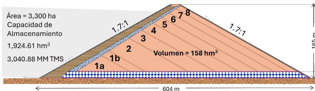
(a) El diseño de la cortina comprende 8 etapas de construcción
